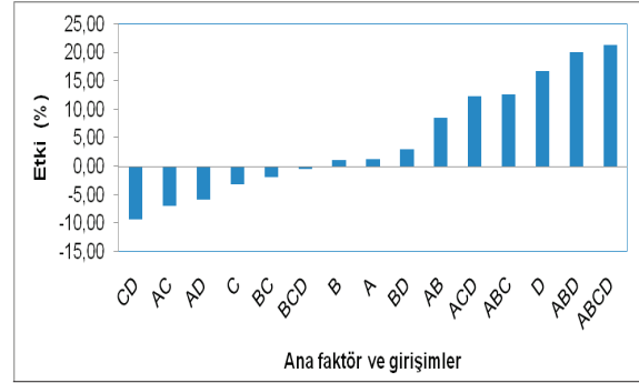
Şekil 4. H 2 O 2 ilavesiyle sitrik asit liçi deneylerinden elde edilen Fe 2 O 3 uzaklaştırma verimlerine etki eden ana faktörler ve girişimler
