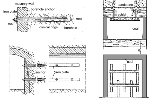
Şekil 4. 1919 yılına ait Königs-hütte kömür madeni için kaya saplama kullanımını gösteren bir çizim (Kovari, 2003b)
