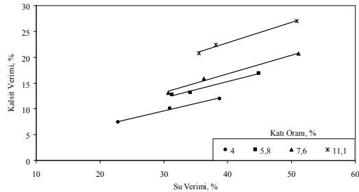
Şekil 9. Katı oranlarının kalsit ve su verime etkisi
