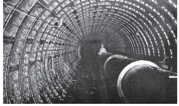
Şekil 10. 1894 yılında Hudson tüneli, New York, Terry Kennedy arşivinden (Brennan, 2004)
